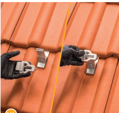
11b Die vertikale Klemmkombination auf die Stütze stecken.
