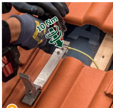
8 ...und die Schraube (10 Nm \pm 0,5 Nm) vollständig anziehen.
