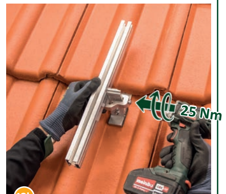
12b Die Klemmkombination mittels Schraube (10 Nm ± 0,5 Nm) festziehen - fertig!
