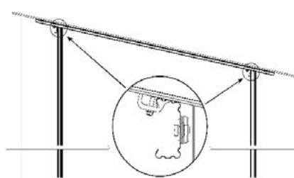
Schraubverbindungen Sparrenträger/Rammprofil
