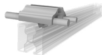
Morsetto parafulmini superiore, altezza d'ingombro molto ridotta per moduli con telaio di 30 mm altezza
